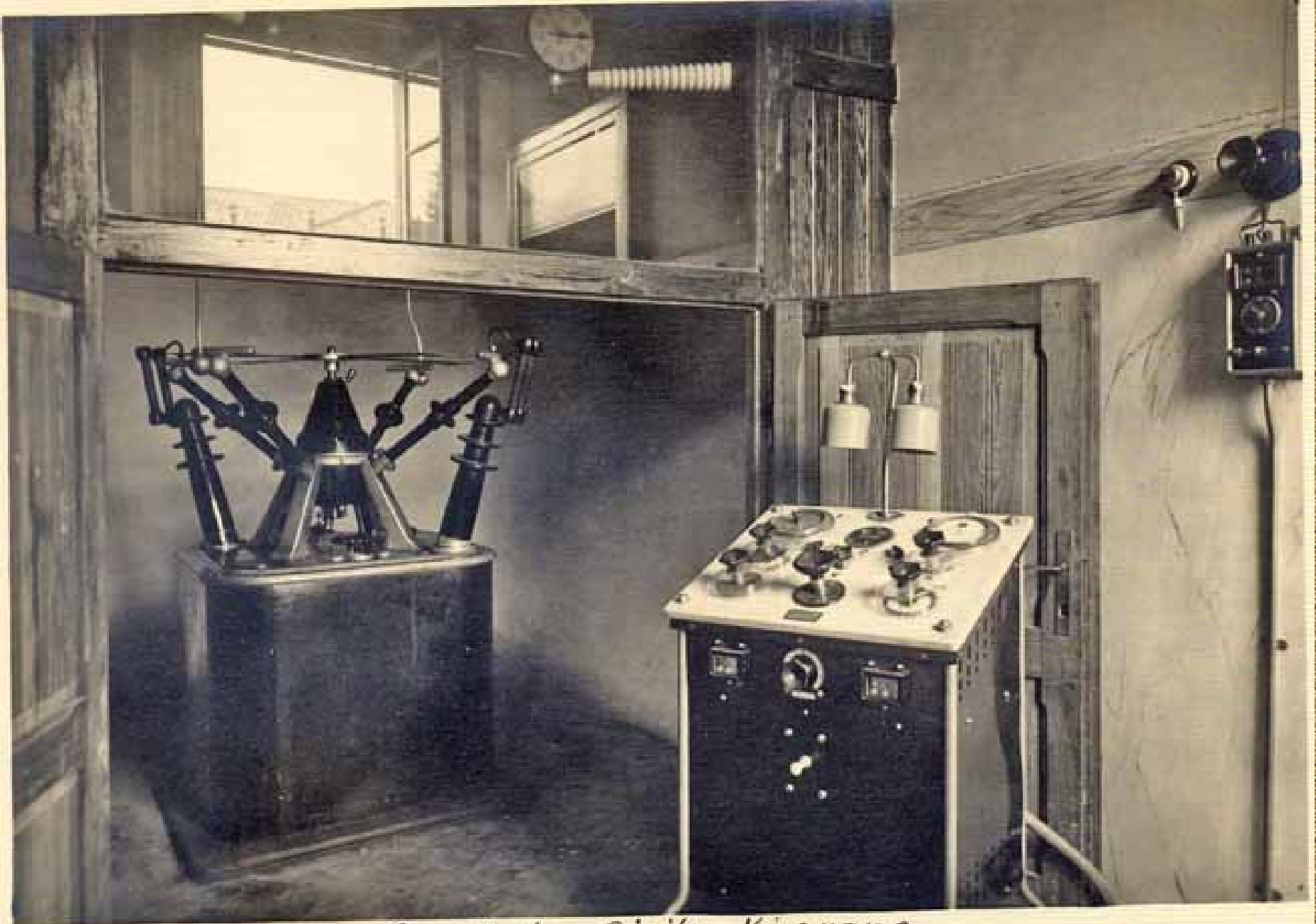
Ospedale Civile Vigevano Gabinetto Radiologico - Trasformatore elettrico e tavolo di comando
